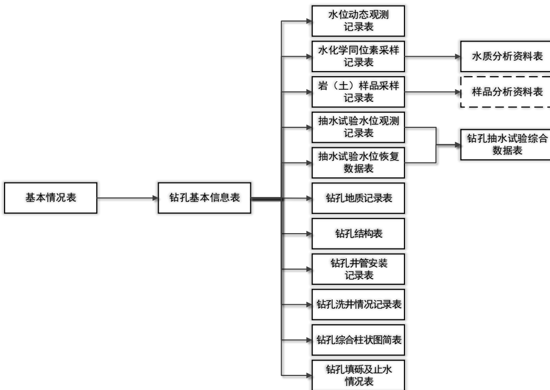
图E.4 水文地质钻探表关联关系
