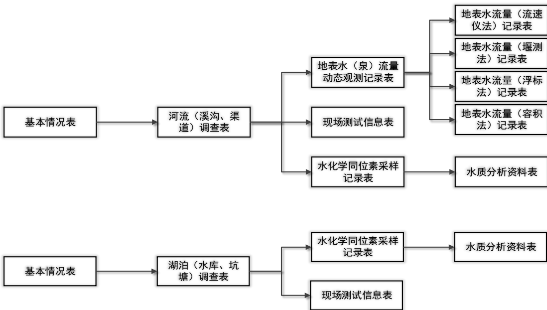
图E. 2 水文地质调查表关联关系
